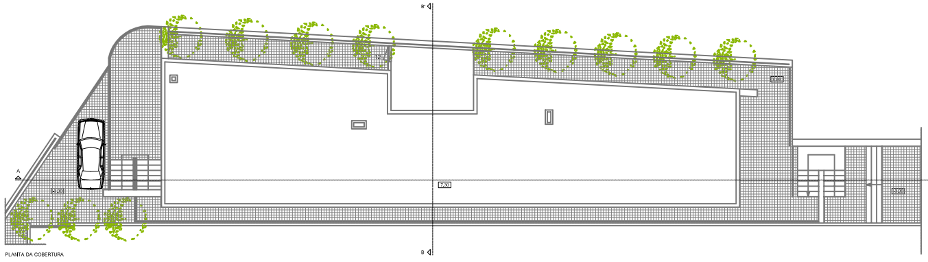
PLANTA DA COBERTURA
