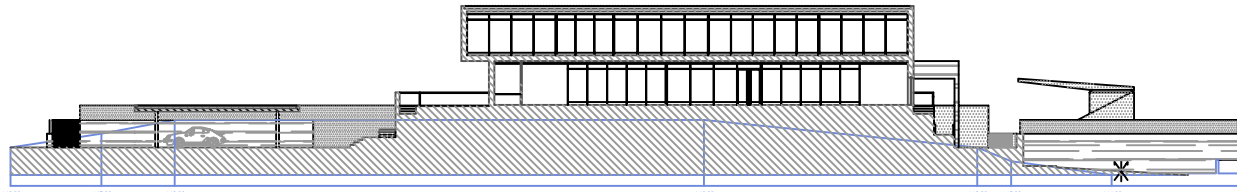
CORTE CC
